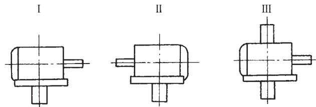
图5 PWS 型减速器及装配型式
