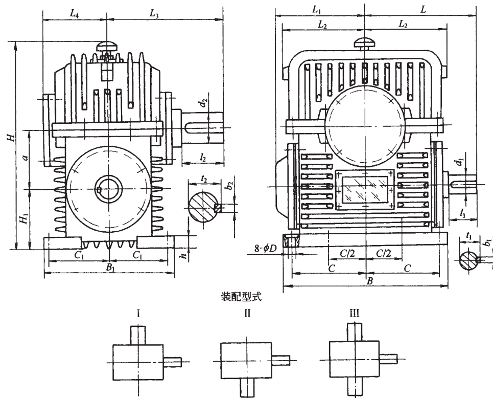
图 2 PWU 型减速器（剖分式）及装配型式
