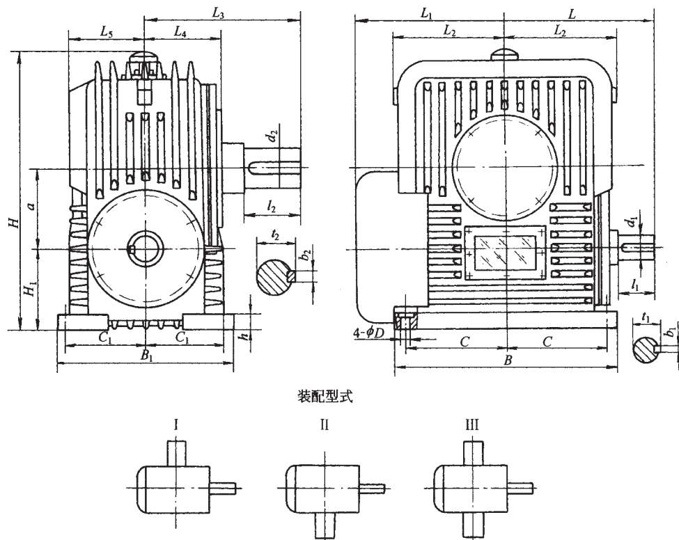
图1 PWU 型减速器（整体式）及装配型式
