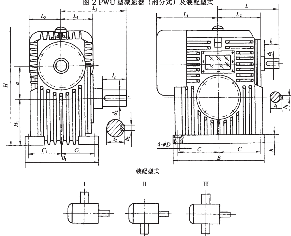
图 3 PWO 型减速器（整体式）及装配型式
