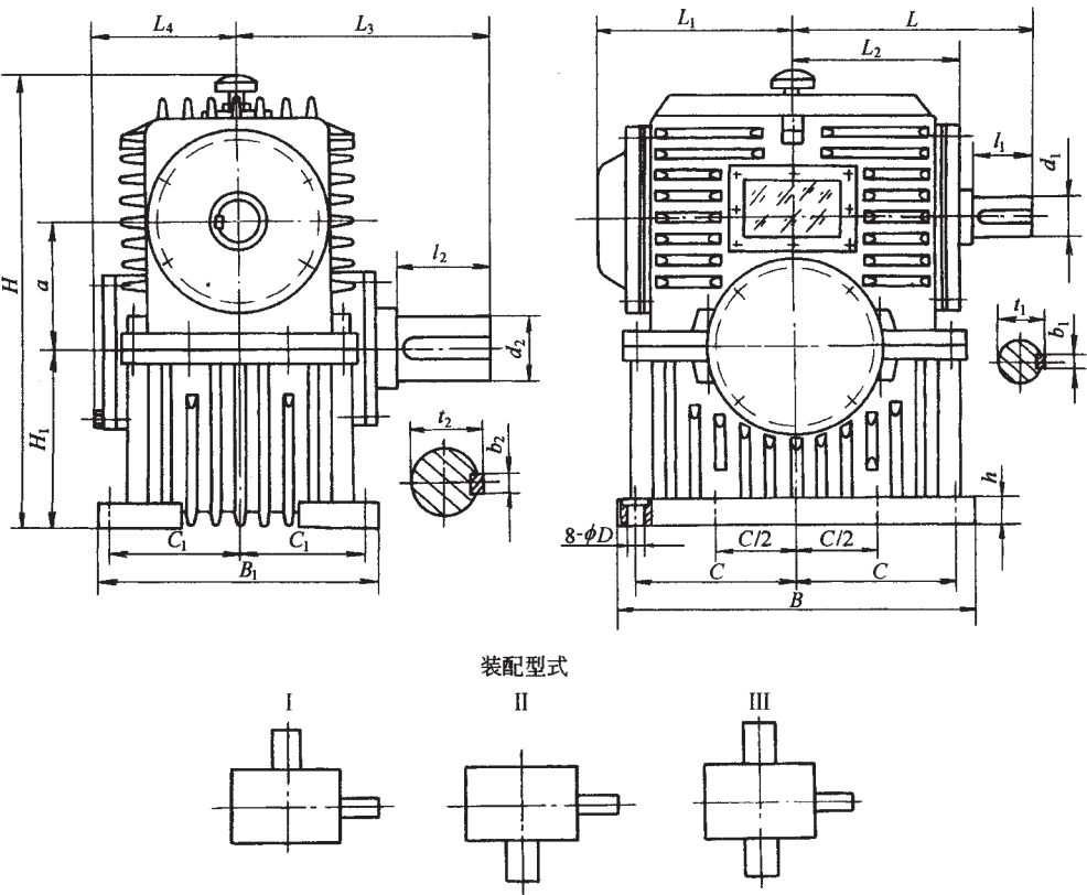
图4 PWO 型减速器 (剖分式) 及装配型式
